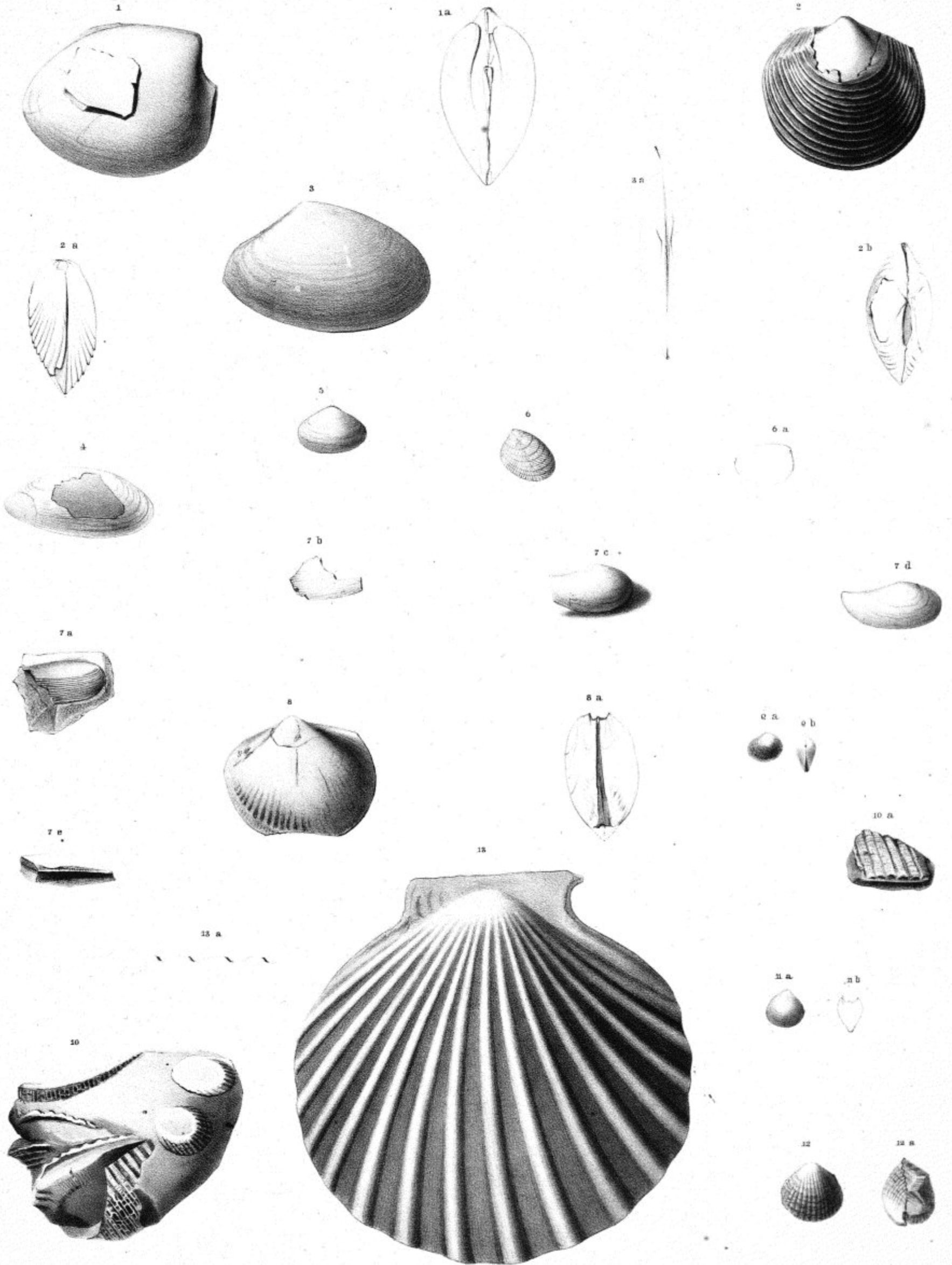
Fig. 1. 1 a. Venus — ? — 2. 2 a, b. Lucina acutilineata. — 3, 3 a. Tellina arcata. — 4. T. emacerata. — 5. T. albaria. — 6, 6 a. Nucula divaricata. — 7 a, b, c, d, e. N. impressa. — 8, 8 a. Pectunculus patulus. — 9 a, b. P. nitens. — 10, 10 a. Arca devincta. — 11 a, b. — ? — 12, 12 a. Cardia subtena. — 13, 13 a. Pecten propatulus.
